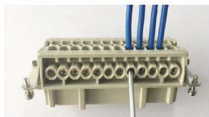
Step 4 连接完成，请拉动线缆以确认线缆确实被弹片夹紧。
