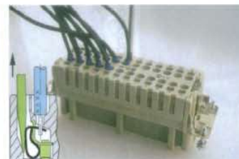
Step 3 取出螺丝起子，弹片收回原位，从而夹紧插入的线缆。
