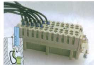
Step 4 连接完成，请拉动线缆以确认线缆确实被弹片夹紧。
